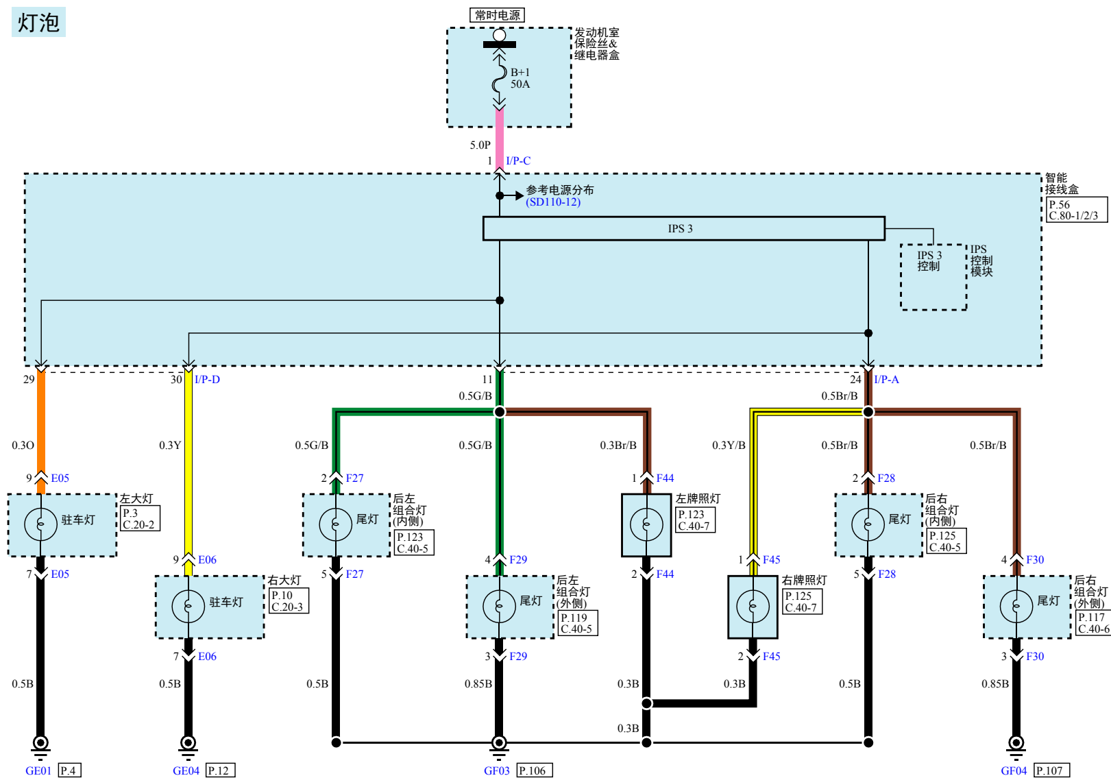
尾灯、驻车灯&amp;牌照灯(2)
