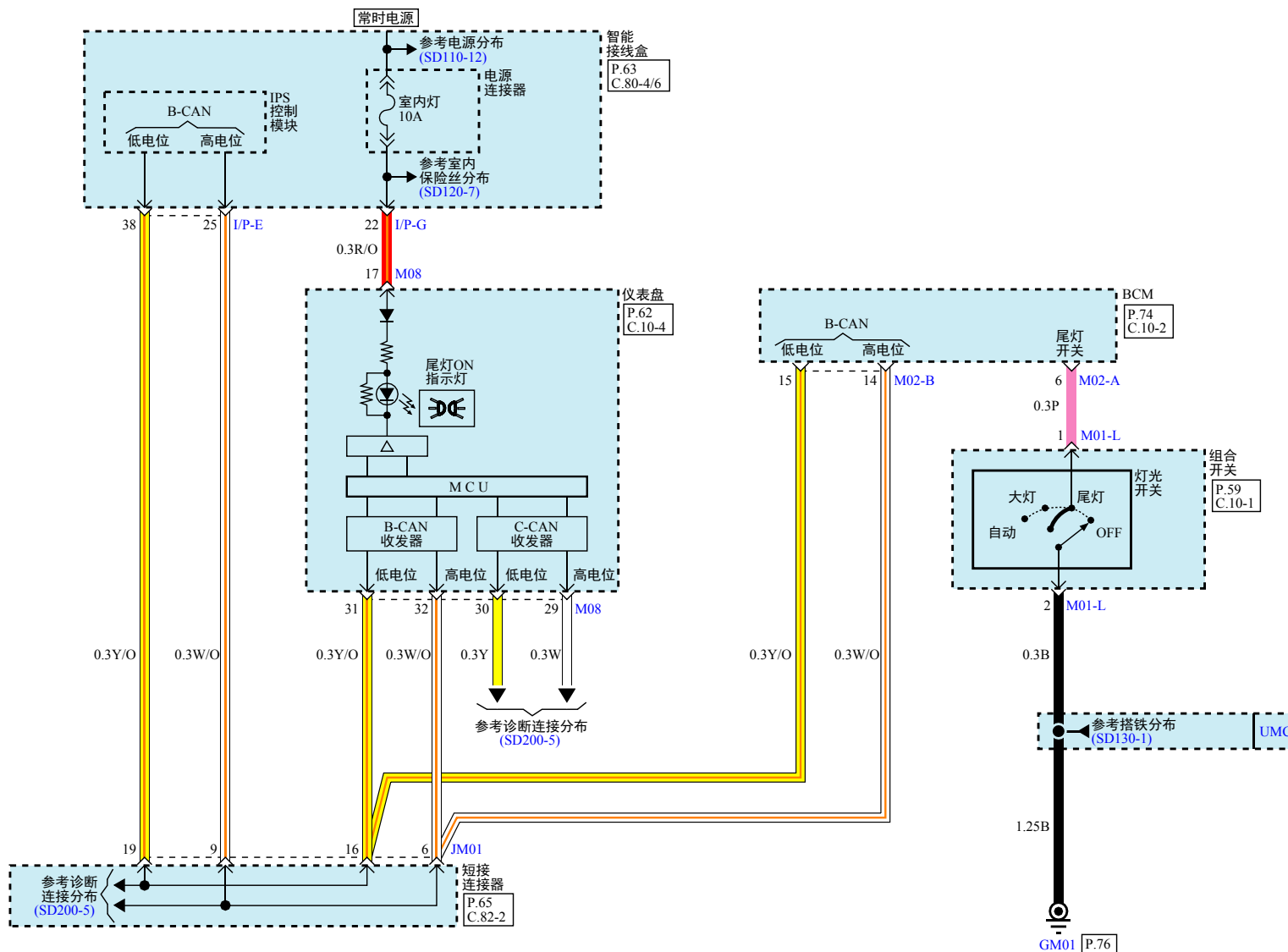
尾灯、驻车灯&牌照灯(1)
